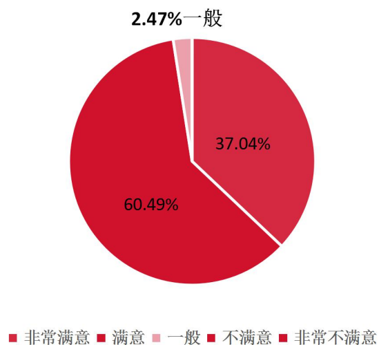
图 3-11 总体满意度
